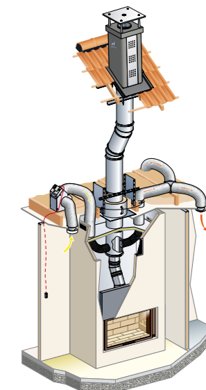
CONFORT+ sur foyer fermé
