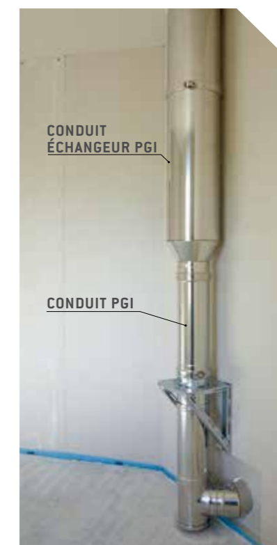
Raccordement à l'arrière du poêle à granulés avant coffrage dans la pièce adjacente
