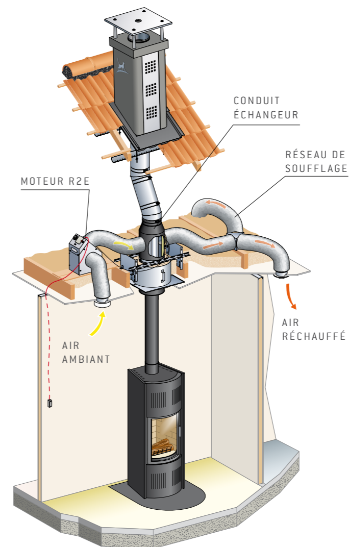
CONFORT+ sur poêle à bois
