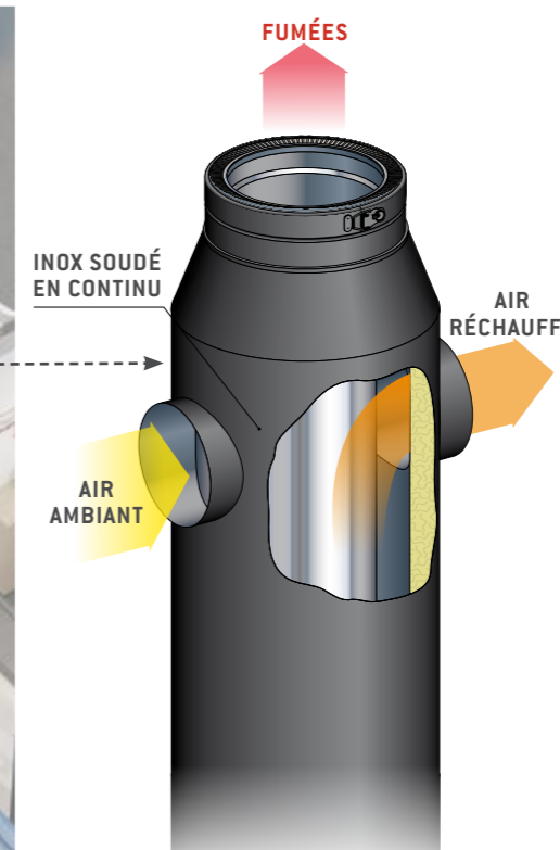
Principe du conduit échangeur
