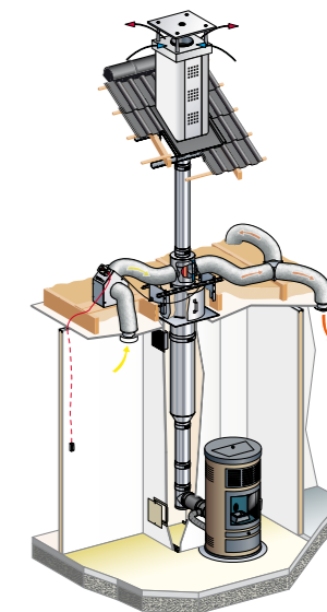
CONFORT+ sur poêle à granulés
