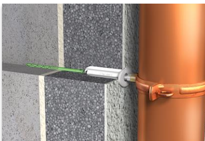
Exemple de fixation d'une descente d'eau pluviale
